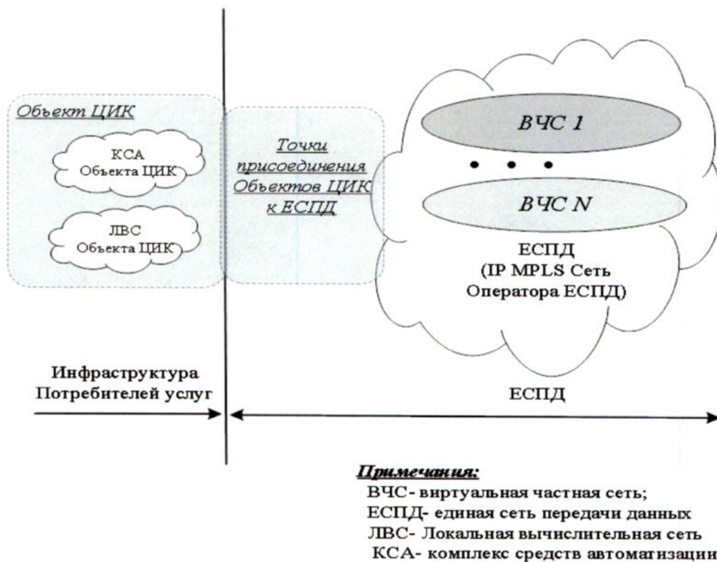
Рис.2. Архитектура Компонента Услуг связи «Предоставление доступа» для Объектов ЦИК
