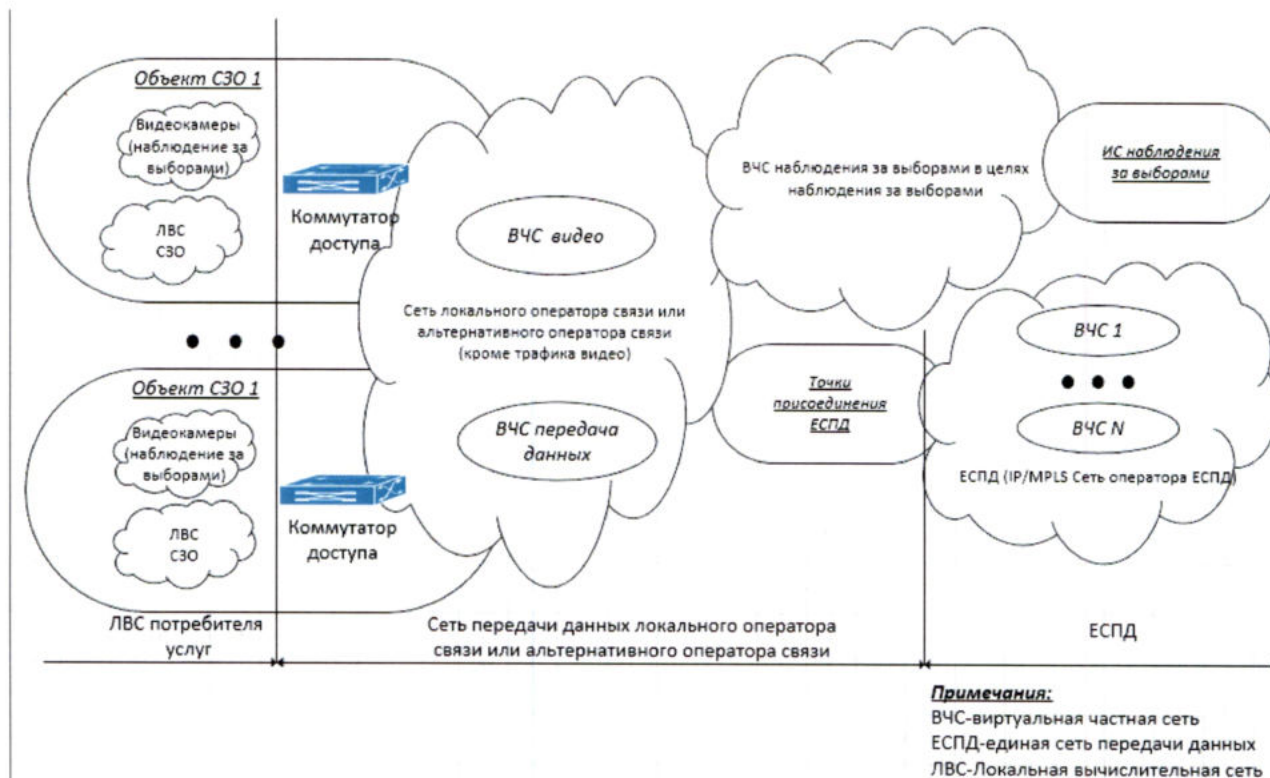
Рис.1. Архитектура Компонента Услуг связи «Предоставление доступа» для СЗО
