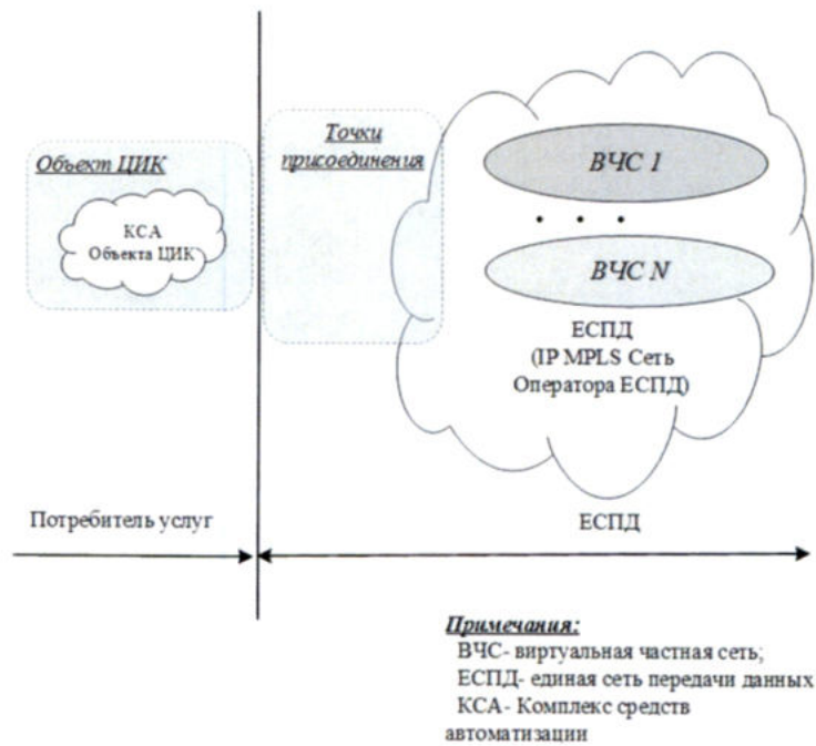
Рис.4.Архитектура Компонента Услуг связи «Передача данных» для Объектов ЦИК.
