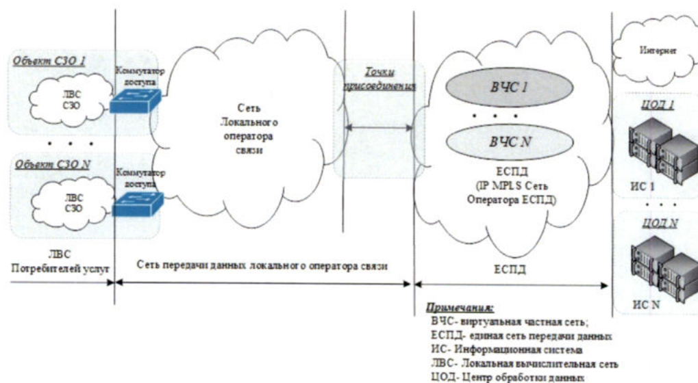
Рис.3. Архитектура Компонента Услуг связи «Передача данных».
